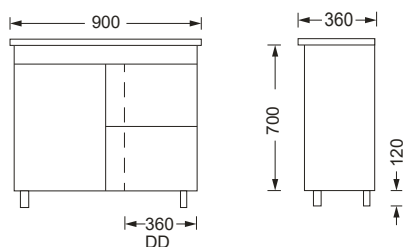
Noah FLS 9036 RH (legs)
