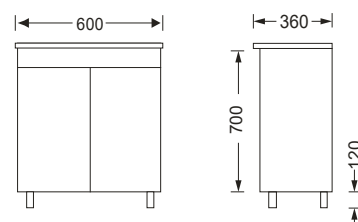
Noah FL 6036 (legs)
